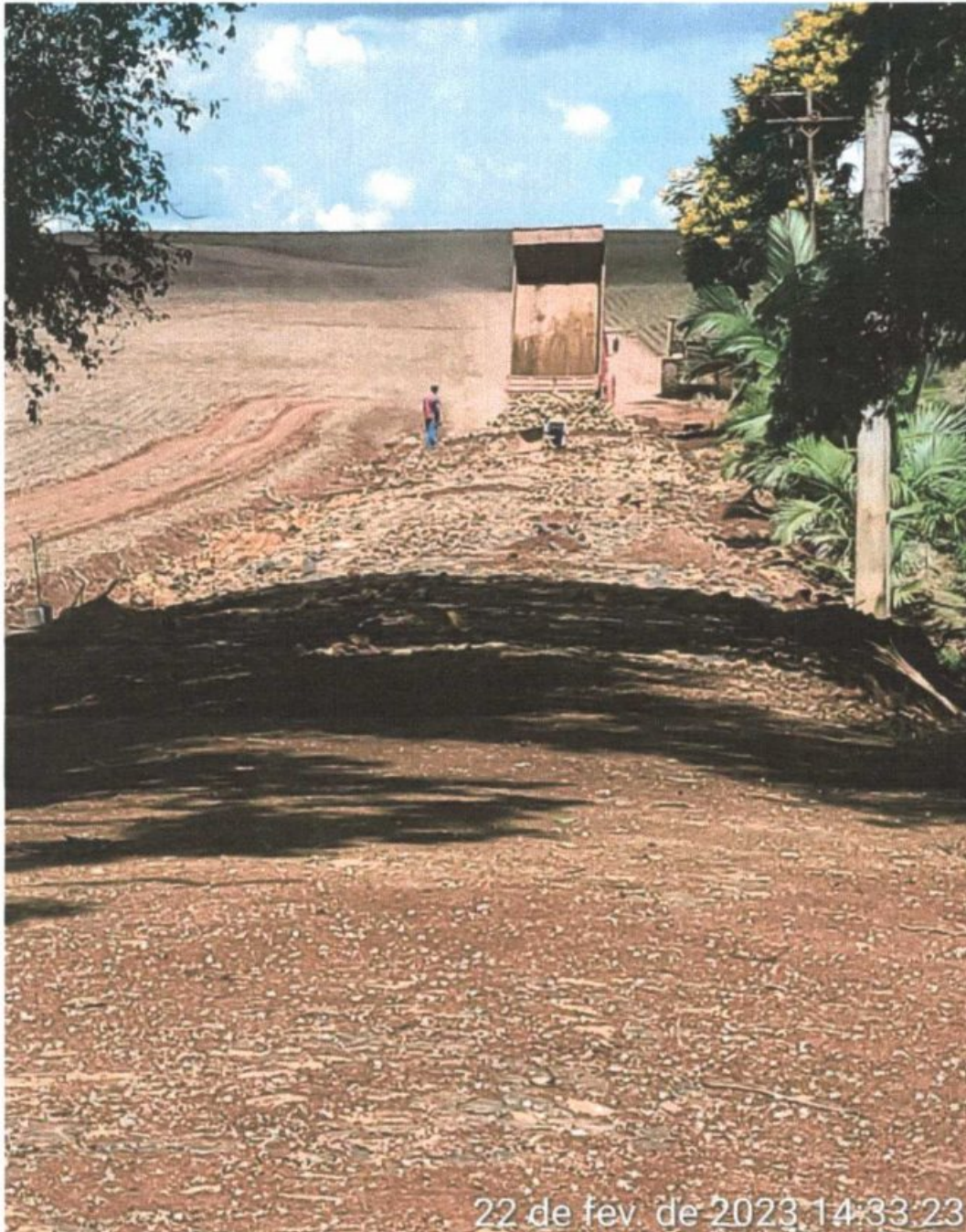
7- ASSENTAMENTO DE PAVIMENTO EM COLCHÃO ARGILOSO DE DESCARREGAMENTO DE MATERIAL.
