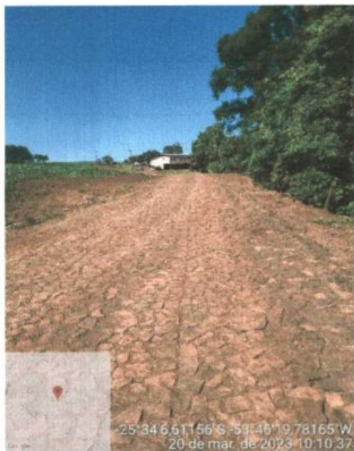
Foto 6-Pavimentação Poliédrica Trecho 01
