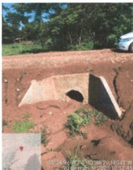
FOTO 4- OBRA DE ARTE CORRENTE TRECHO 01
