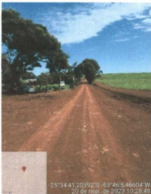
Foto 12-Pavimentação Poliédrica Trecho 04
