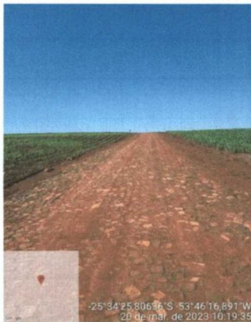
Foto 9-Pavimentação Poliédrca Trecho 03
