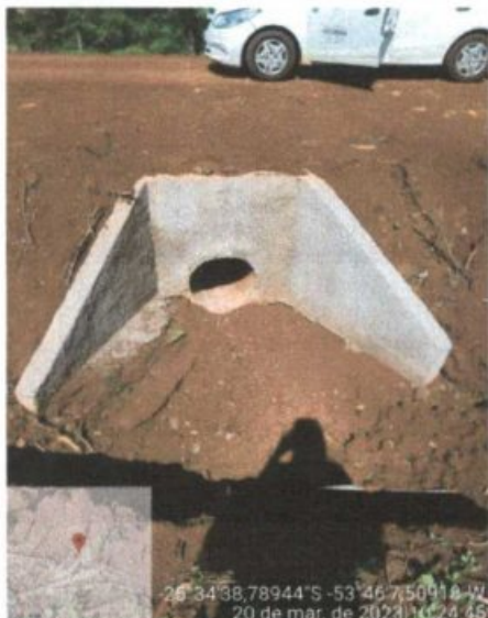
FOTO 4- OBRA DE ARTE CORRENTE TRECHO 04
